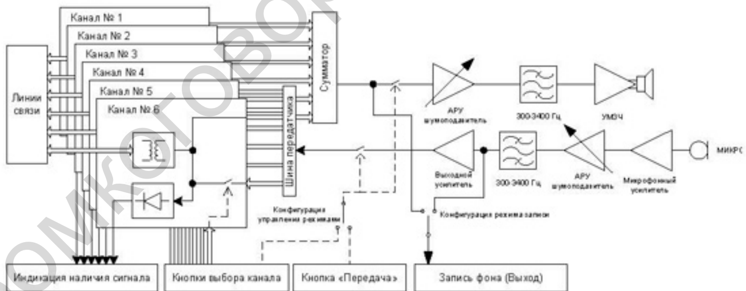
Рис. 3. Структурная схема ПГС-5-6У.
